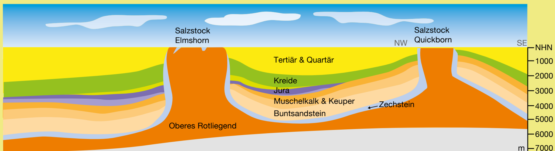
◀ Profilschnitt (schematisch, nicht überhöht) durch einen Teil Südholsteins mit den Salzstöcken Elmshorn und Quickborn. Das Salz ist in den Schichtfolgen des Zechstein und des Oberen Rotliegend enthalten. (Zeichnungsvorlage aus "fossilien, journal für erdgeschichte" 3/2015, Quelle & Meyer Verlag)
